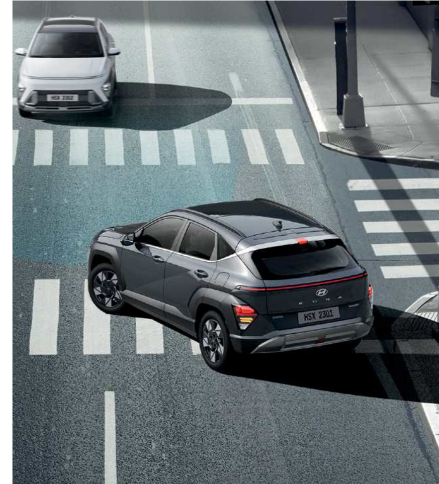
בלימה אוטונומית במצבי חירום (FCA-JT) מערכת אקטיבית המתריעה מפני סכנת התנגשות. במידה וסכנת ההתנגשות עולה לאחור ההתרעה, המערכת תבצע בלימת חירום אוטומטית. המערכת כוללת זיהוי כלי רכב, דו גלגלי ותנועה חוצה בצומת מכל הכיוונים.
